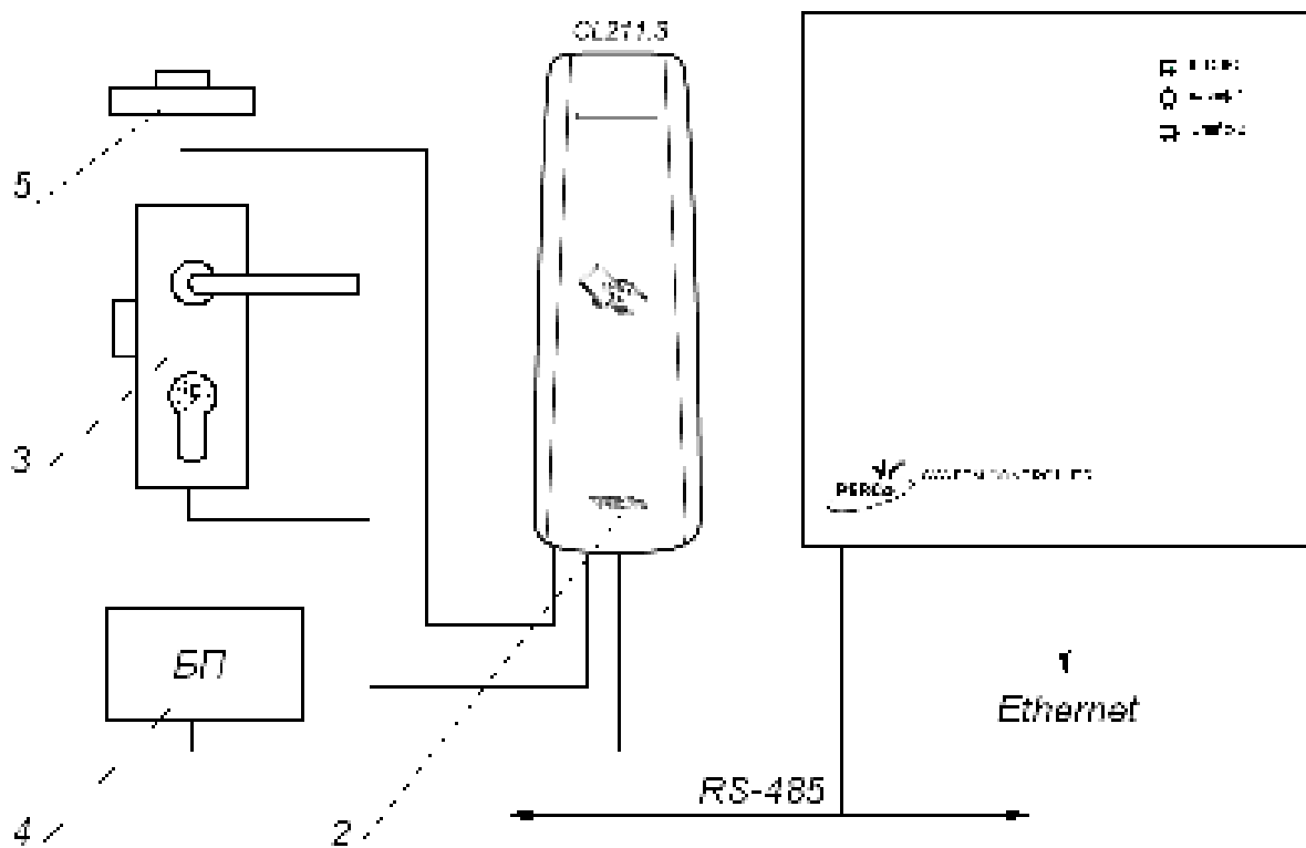
Рисунок 1. Функциональная схема
