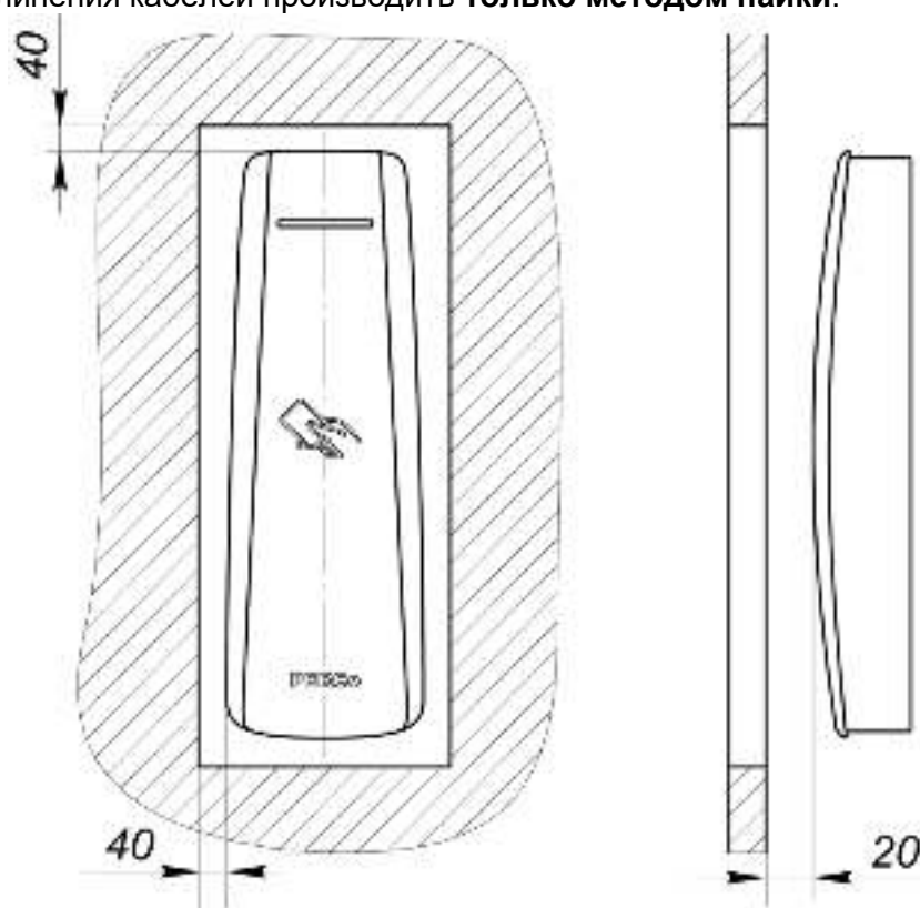
Рисунок 2. Установка контроллера за металлической поверхностью
