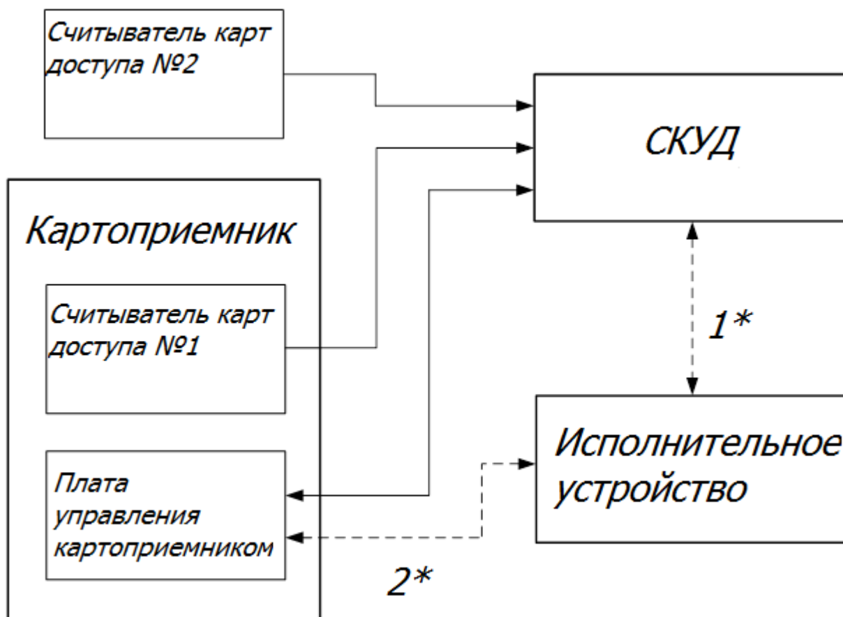
Рисунок 18 – Структурная схема №1
