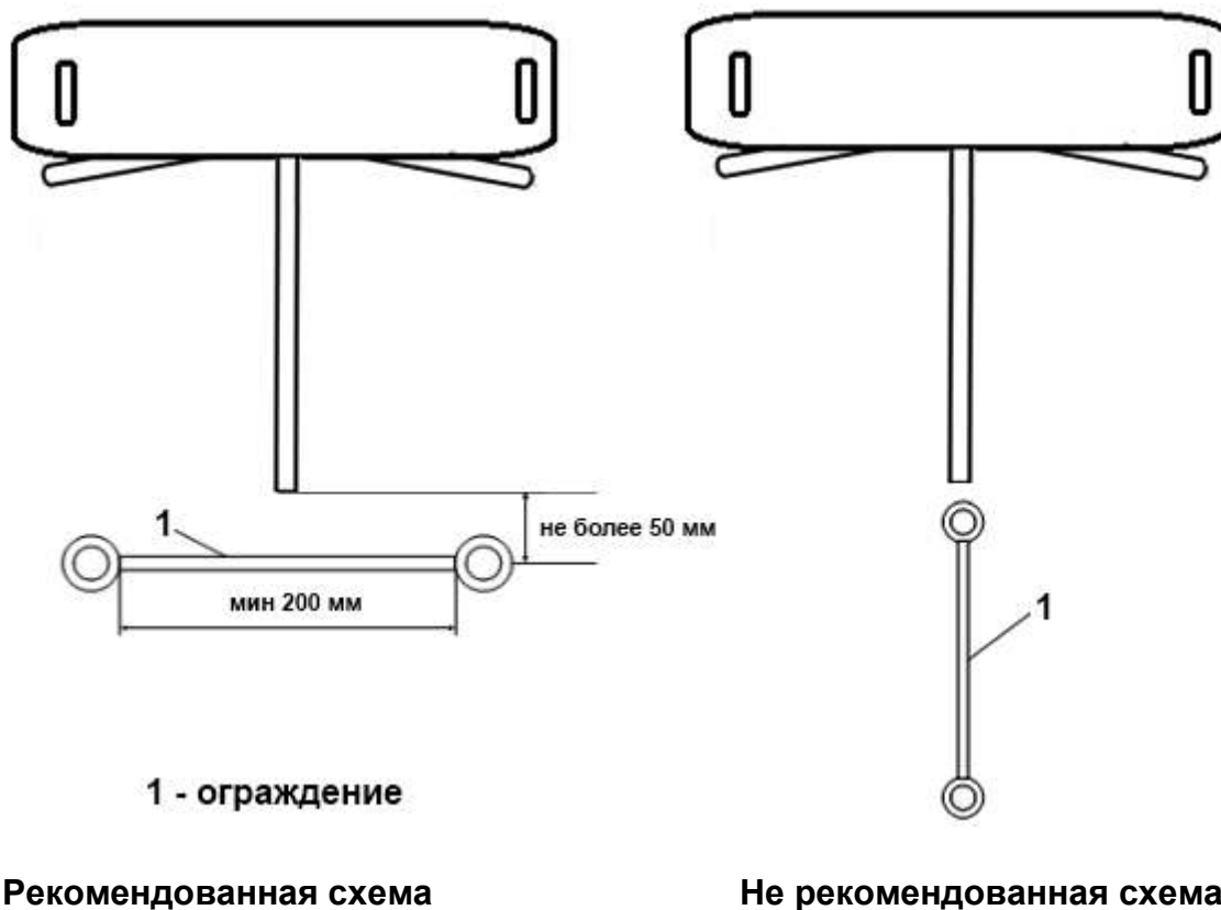
Рисунок 3 – Организация зоны прохода турникета.
