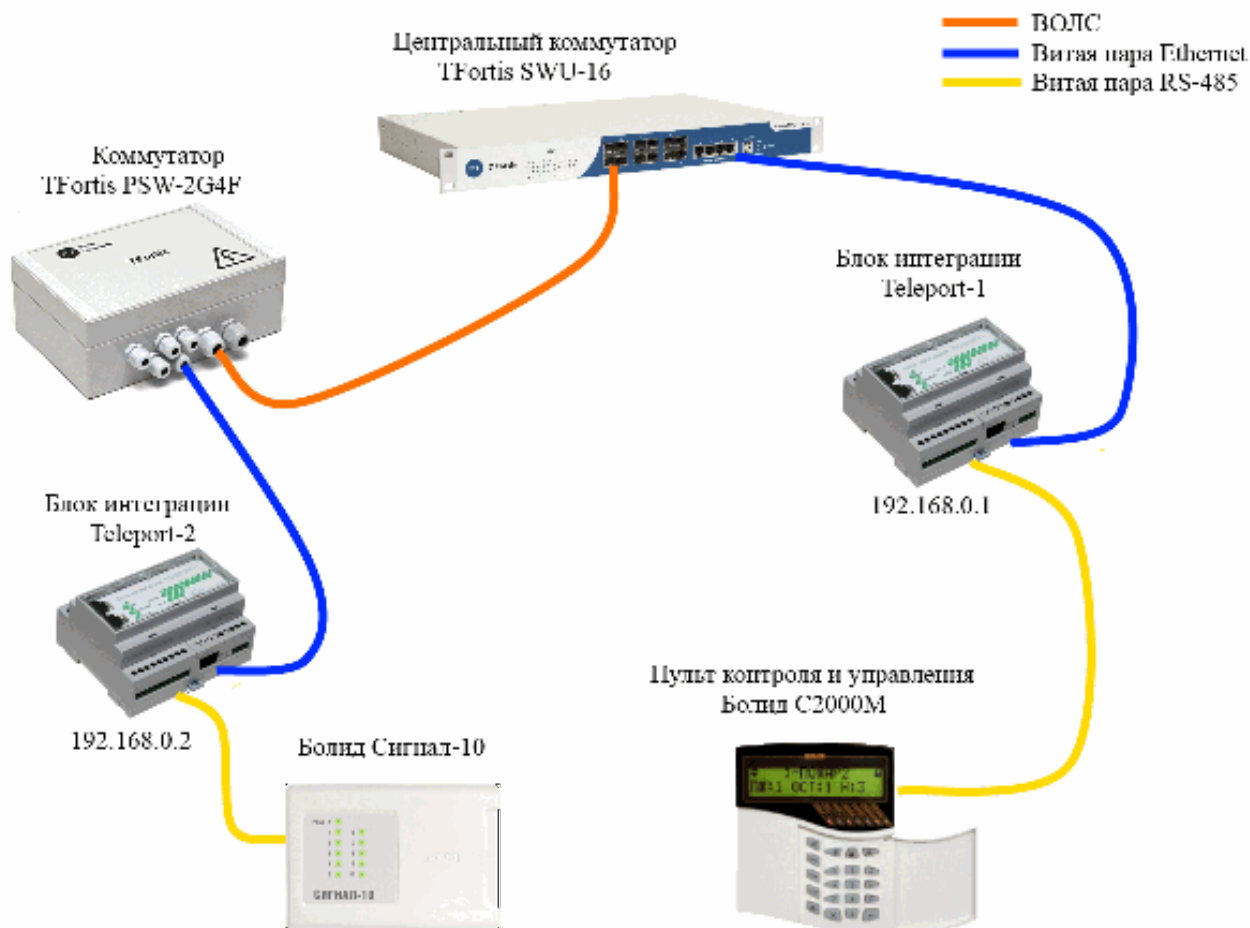
Рис. 2. структура системы
