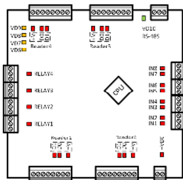
Индикаторы модуля расширения ST-NB441D
