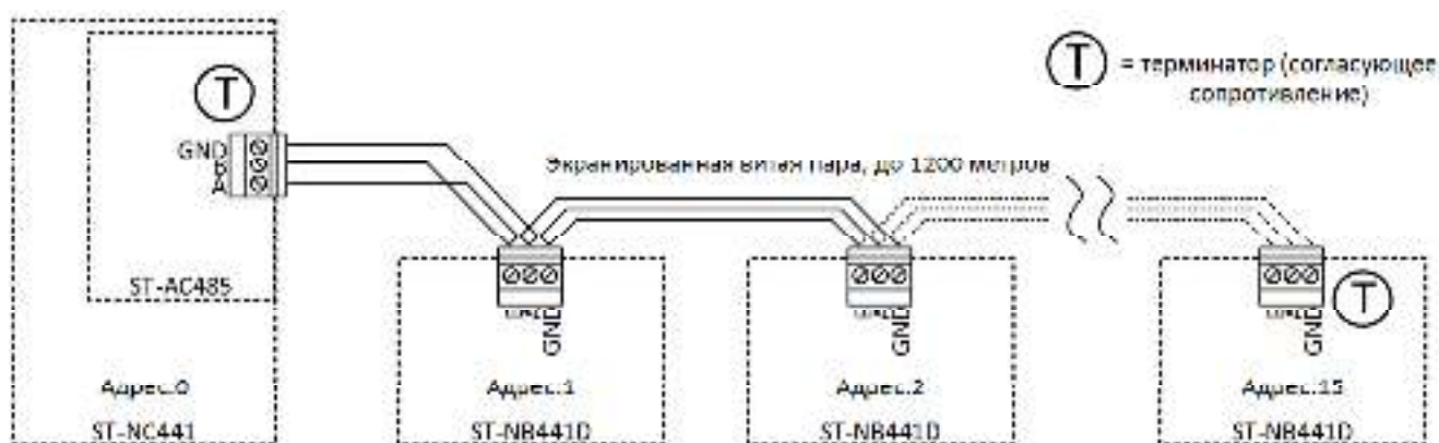
Расположение переключек на модуле расширения ST-NB441D
