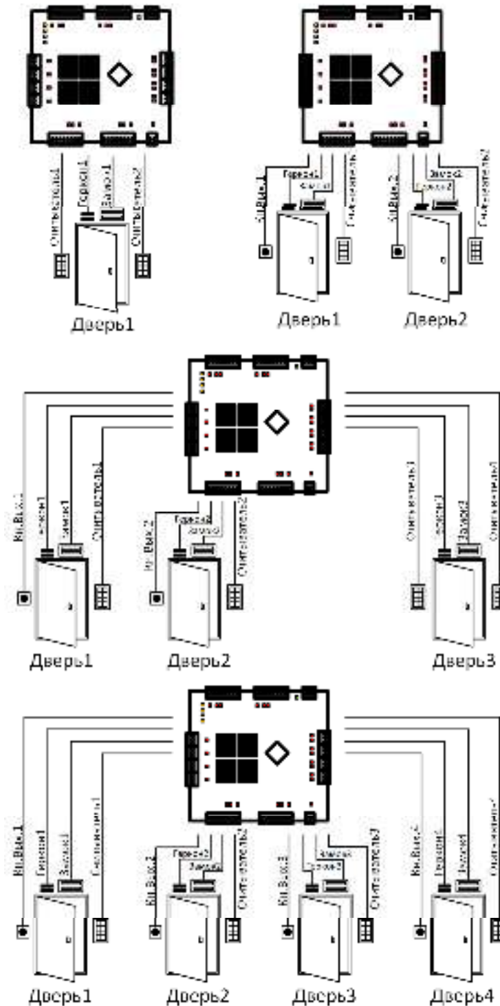
Примеры конфигурации модуля ST-NB441D
