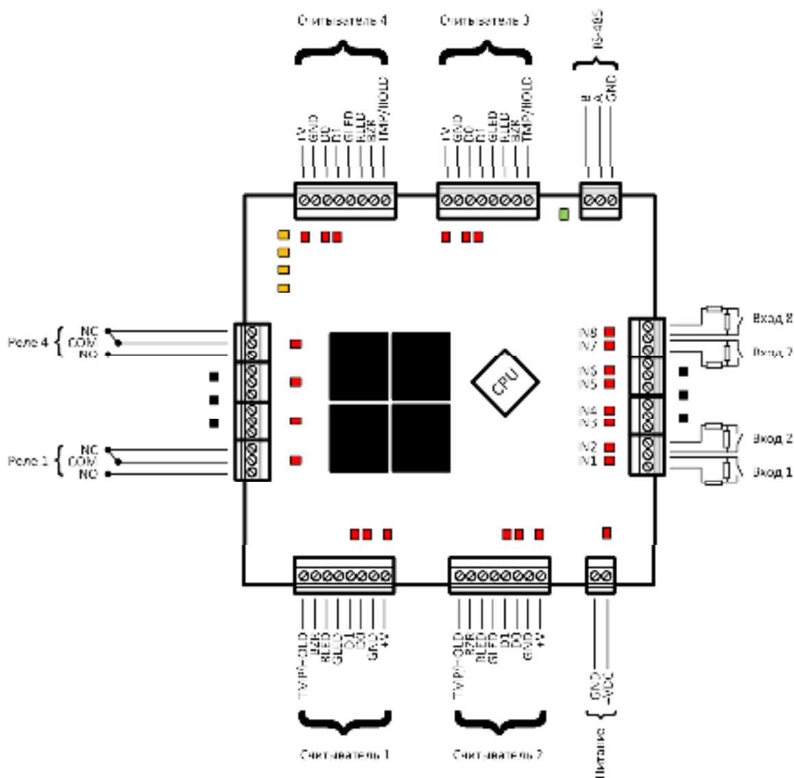
Назначение контактов модуля расширения ST-NB221D
