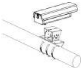
Рисунок 2-6 Установка корпуса
